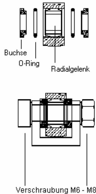
Einbau mit Radialgelenken
